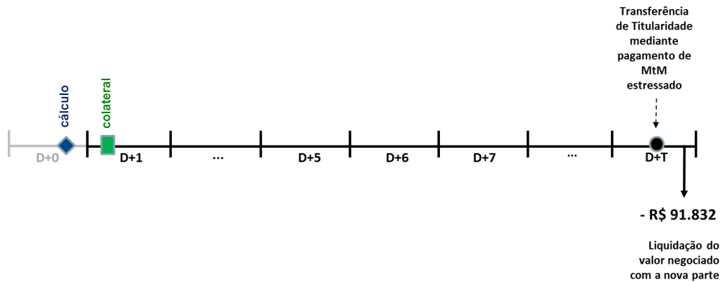
Figura 7.70 - Projeção de liquidação do valor do swap
